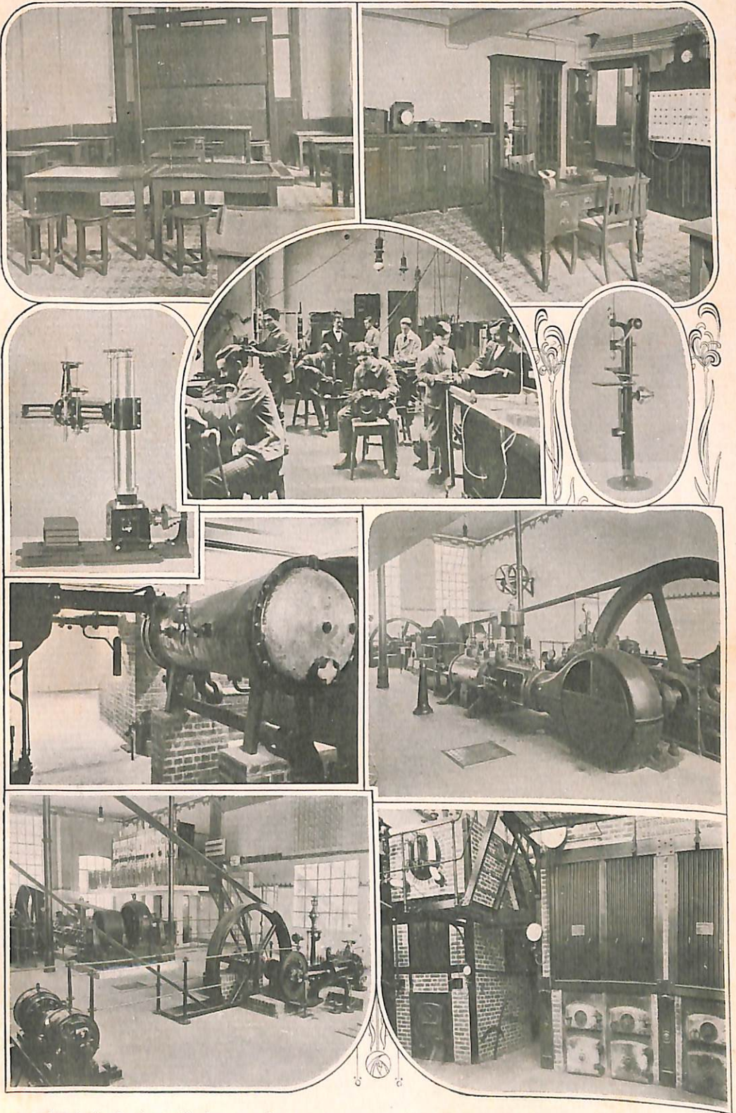
1. Laboratorio de electrotécnica. — 2. Laboratorio de electrotécnica. — 3. Agujereadora radial (construida en la escuela). — 4. Taller de Electricidad. — 5. Taladradora rápida (construida en la escuela). — 6. Sótano de la central eléctrica, condensador de superficie. — 7. Central eléctrica (motores). — 8. Central eléctrica (motores). — 9. Central eléctrica (calderas).
